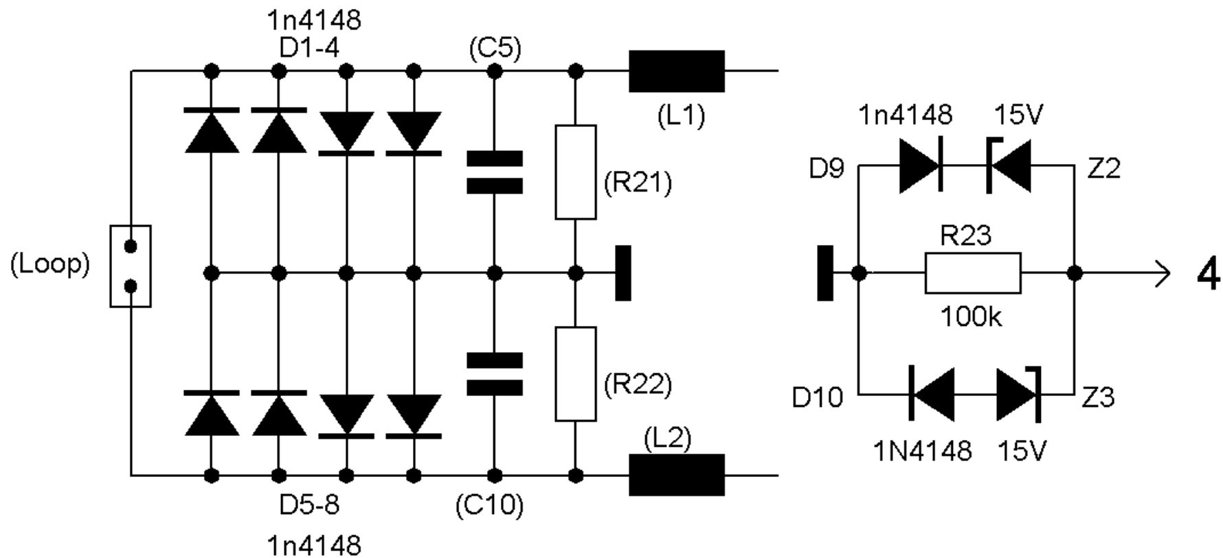
LZ1AQ RXloop Amp. overspanning beveiliging.
